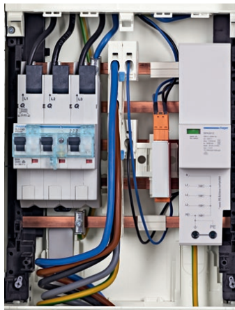
Abbildung 4: Spannungsabgriff aus NAR (ungezählt) mit Einspeiseadapter und Sicherungsbox (25 kA) auf Geräteträger
