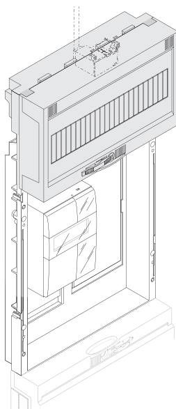
Abbildung 1: RfZ bei BKE-I mit 12 PLE (Neubau)
