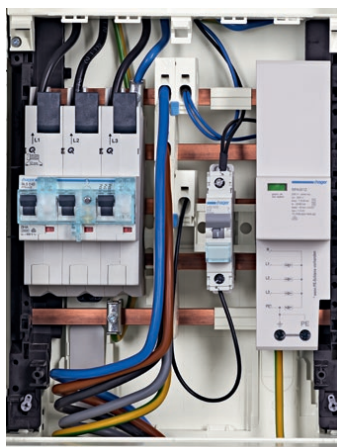
Abbildung 5: Spannungsabgriff aus NAR (ungezählt) mit Einspeiseadapter und LS-Schalter (25 kA) auf Geräteträger
