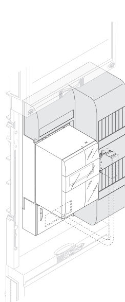
Abbildung 2: RfZ bei 3-Punkt mit BKE-AZ (Bestand)
