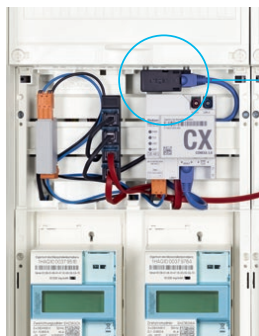
BKE-I-Kassette mit Sicherungsbox und RJ45-Buchse
