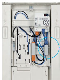
BKE-AZ-Adapter mit Spannungsabgriffen, Sicherungsbox und RJ45-Buchse
